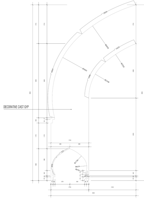
ID 02 MEHRAB DETAIL (02) 1:20
